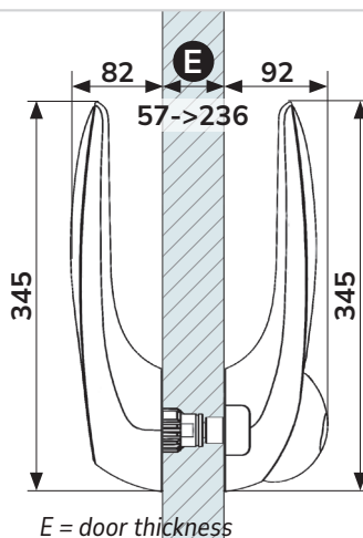
Semi-inset door
